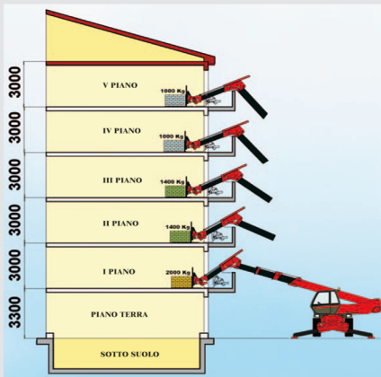
MRT 2440 EPS POSIZIONAMENTO DEL CARICO ALL'INTERNO DELL'EDIFICIO CON BALCONI
